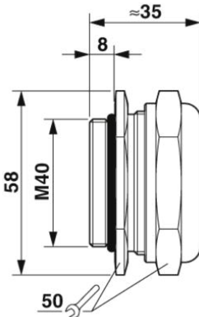
Esquema de dimensiones
