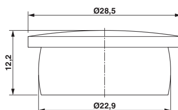
Esquema de dimensiones
