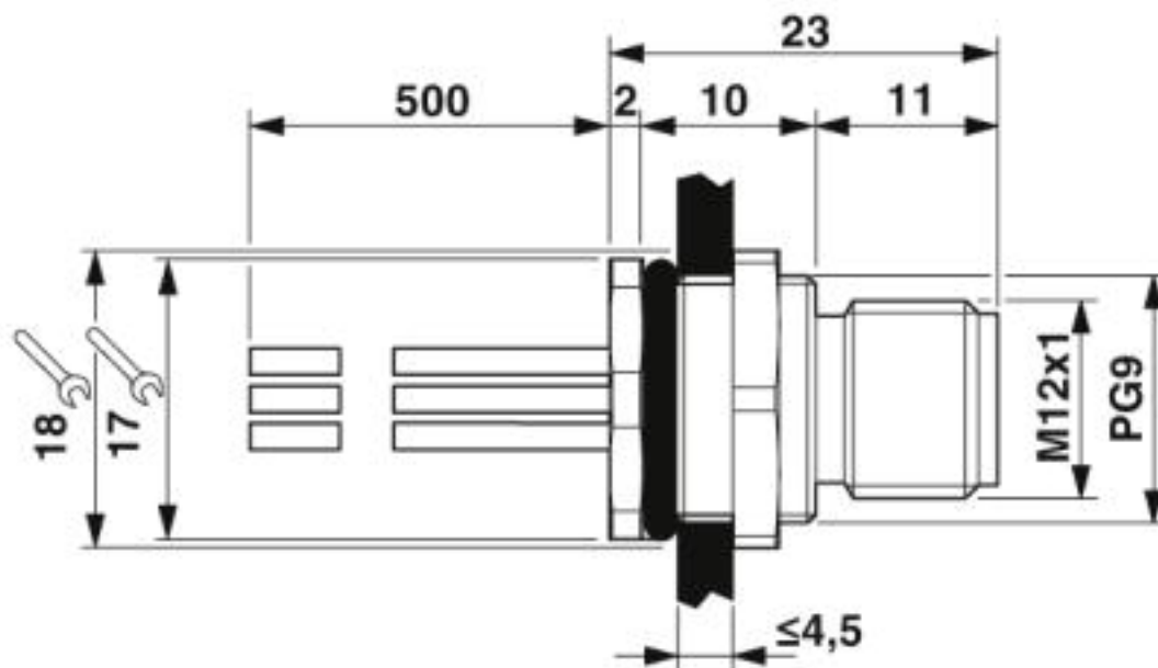
Macho de montaje incorp. M12
