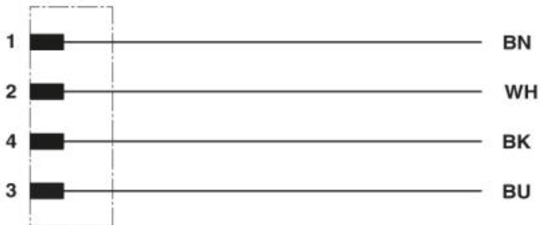
Diagrama eléctrico
