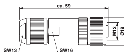
Conector hembra M12 x 1, recto, apantallado
