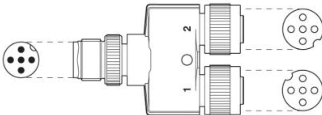
Plano esquemático
