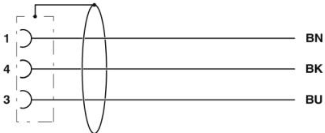
Diagrama eléctrico
