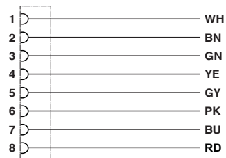
Diagrama eléctrico
