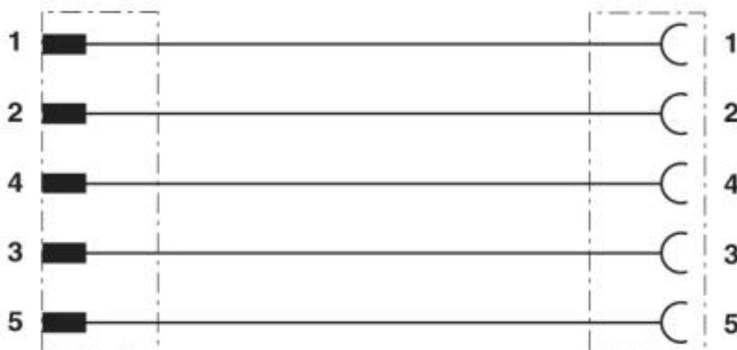
Diagrama eléctrico
