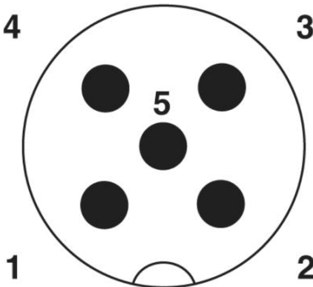
Plano esquemático
