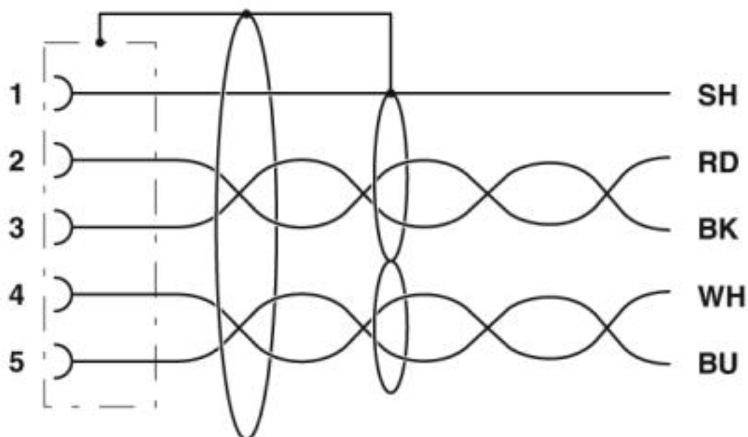
Diagrama eléctrico
