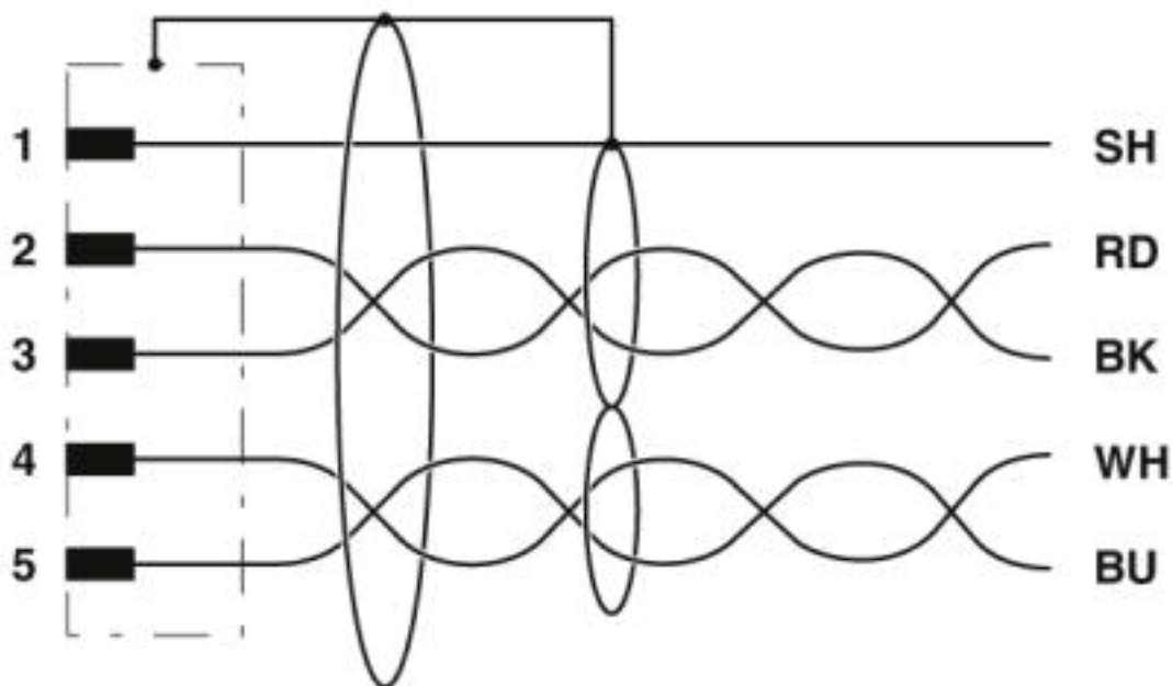
Diagrama eléctrico
