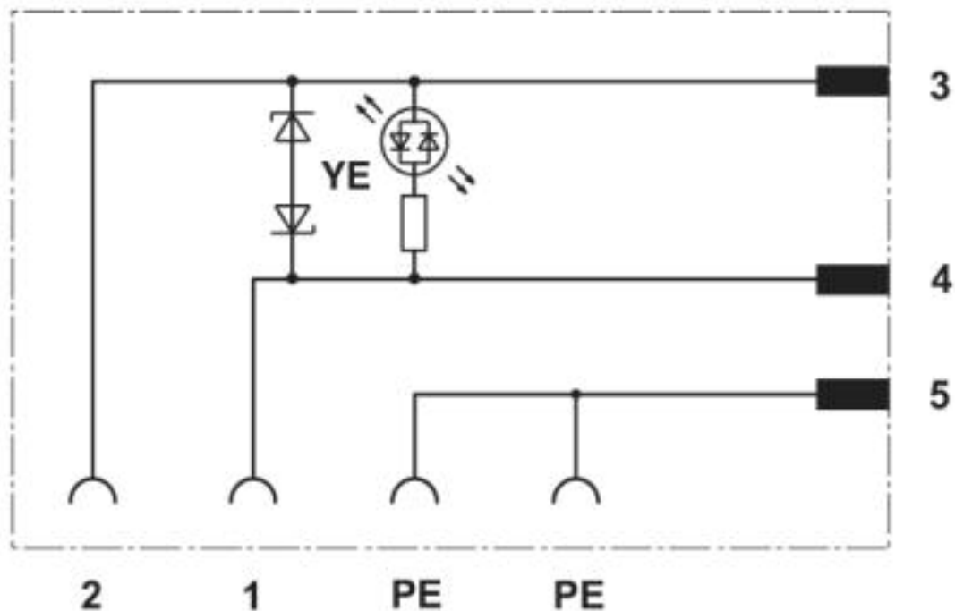
Diagrama eléctrico
