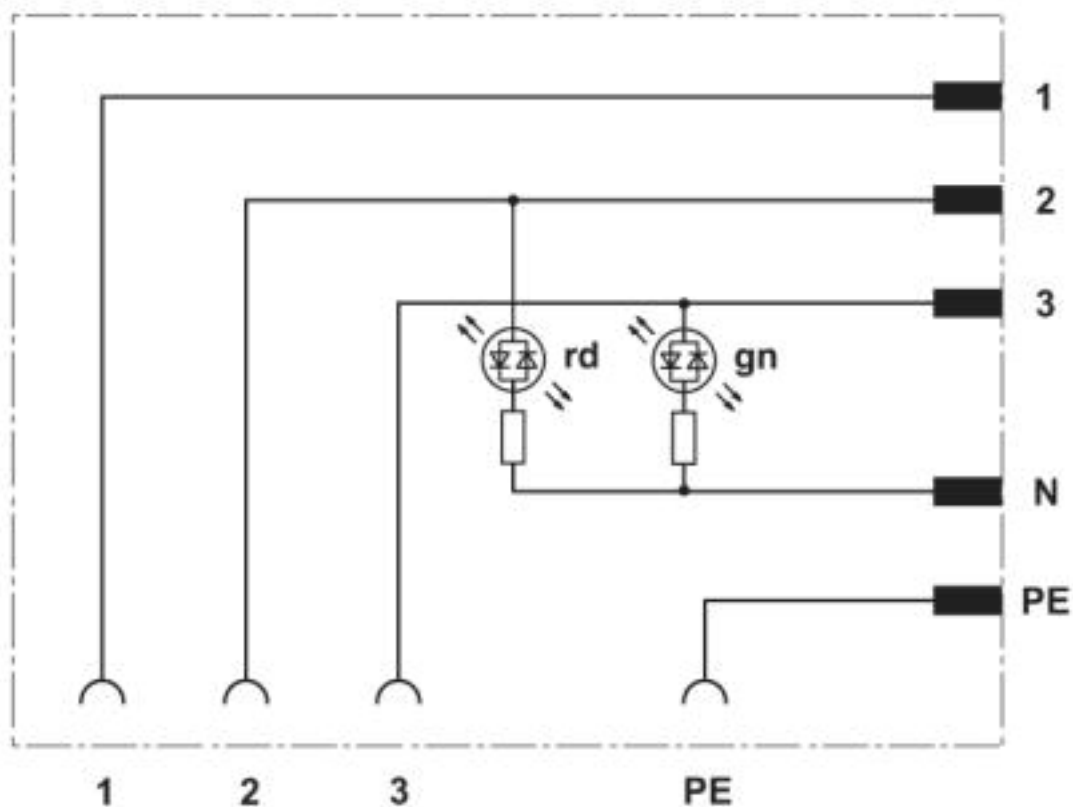
Diagrama eléctrico
