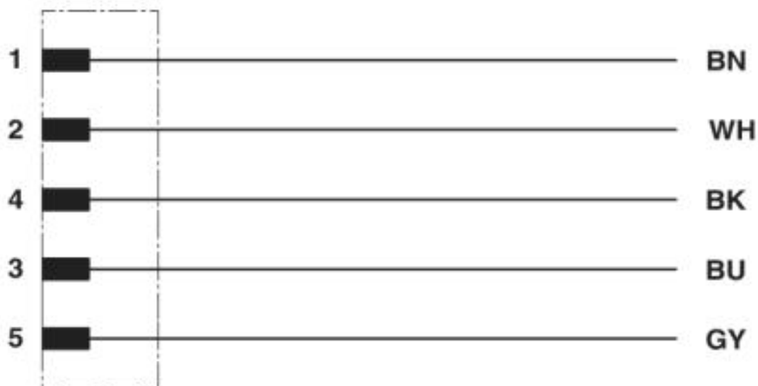
Diagrama eléctrico
