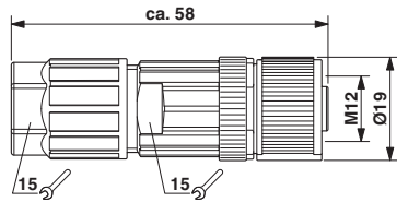
Esquema de dimensiones
