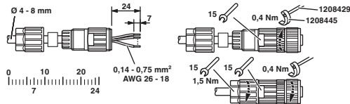
Dibujo funcional
