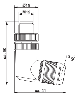
Conector macho SPEEDCON M12, acodado, apantallado
