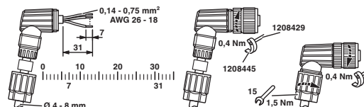
Dibujo funcional
