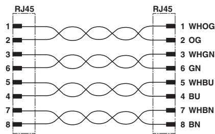
Diagrama eléctrico
