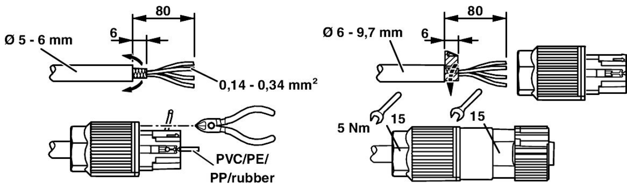
Dibujo funcional
