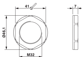
Esquema de dimensiones
