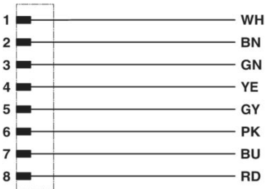
Diagrama eléctrico
