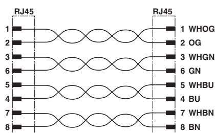
Diagrama eléctrico
