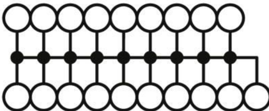
Diagrama eléctrico
