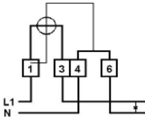
Medidor de 2 hilos (1 sistema), versión DIN
