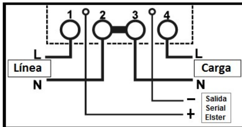
Diagrama de Conexión:
