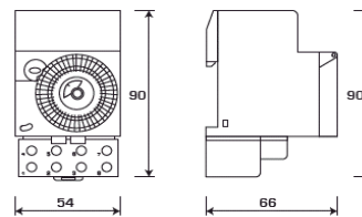
Dimensiones (mm)
