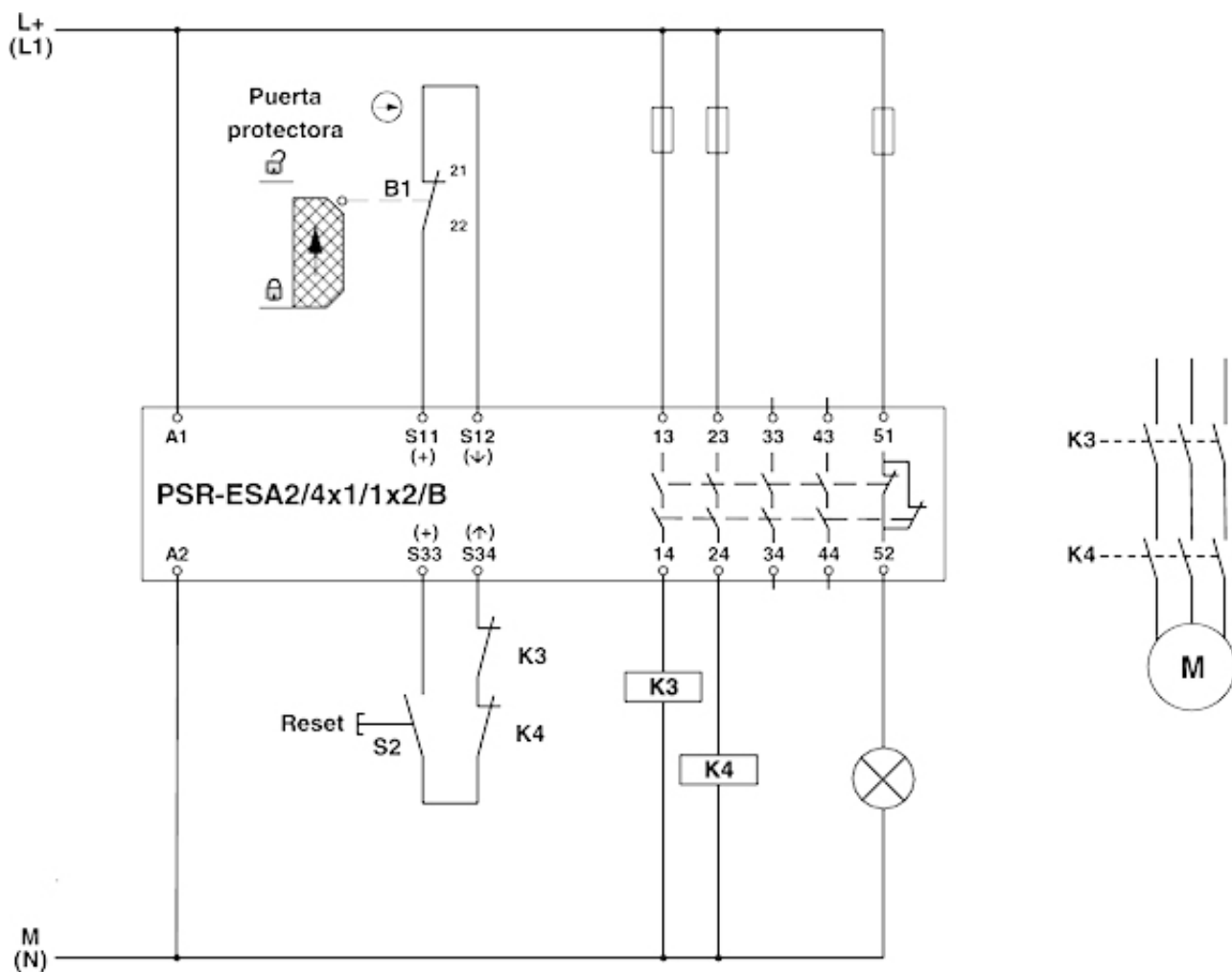
Diagrama eléctrico
