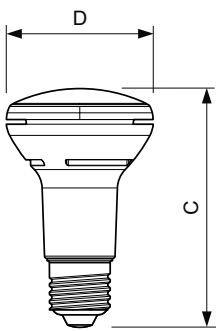
R63 CL 230V 6W-50W 36D 2700K E27 Dim
