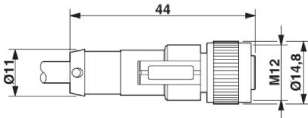
Conector hembra M12 x 1, recto
