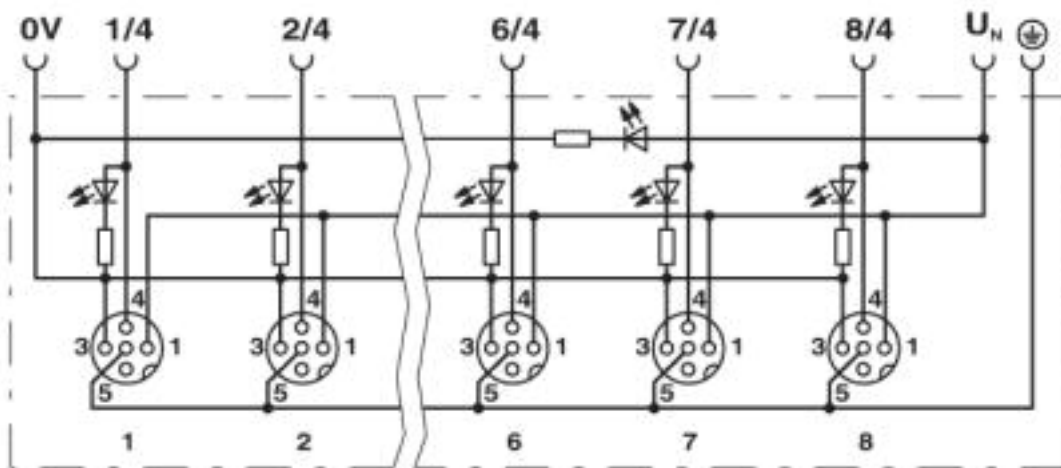
Diagrama eléctrico
