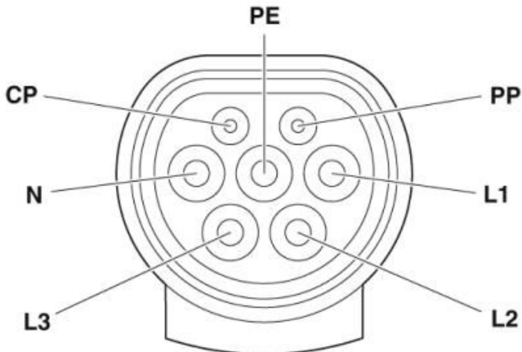
Plano esquemático
