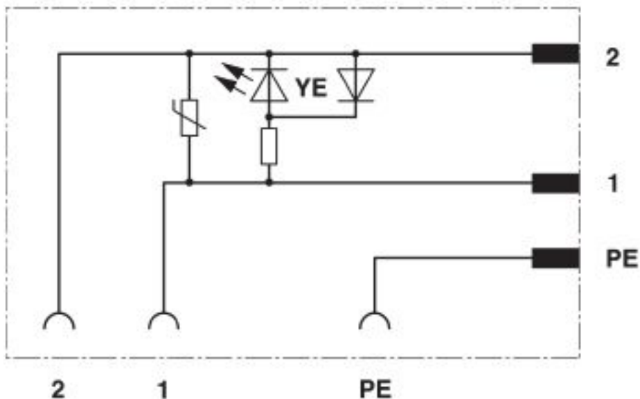
Diagrama eléctrico
