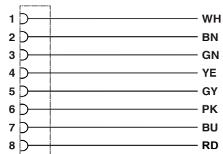
Diagrama eléctrico
