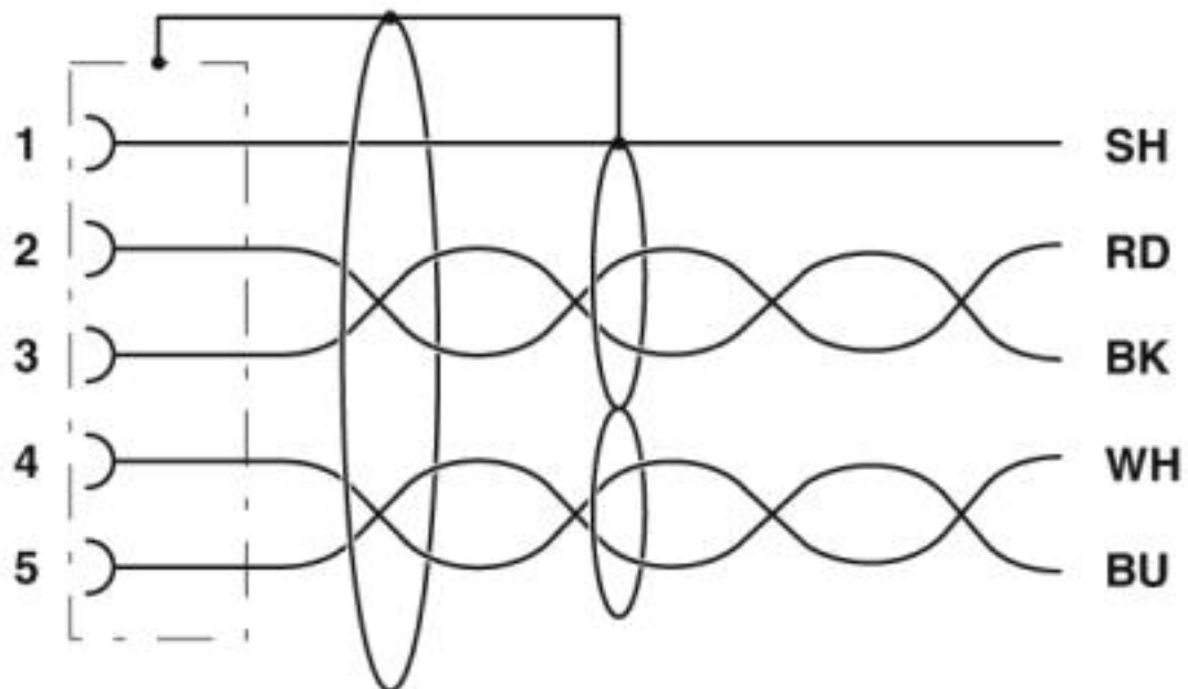
Diagrama eléctrico
