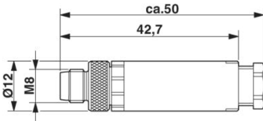
Conector macho M8 x 1, ejecución recta
