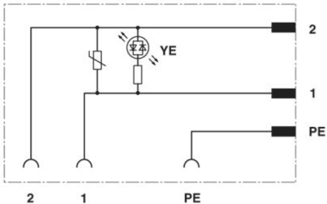
Diagrama eléctrico
