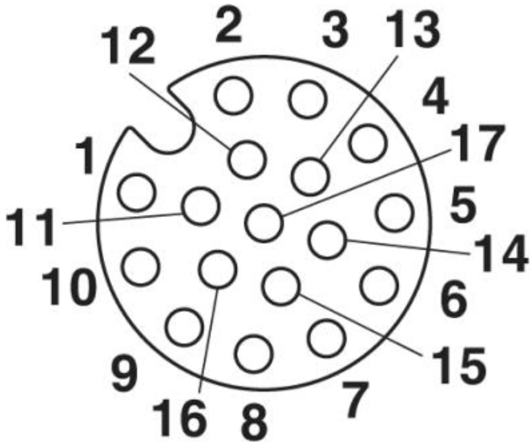
Esquema de polos del conector hembra M12, 17 polos, vista de la cara de hembras
