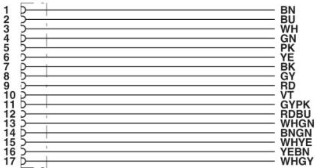
Diagrama eléctrico
